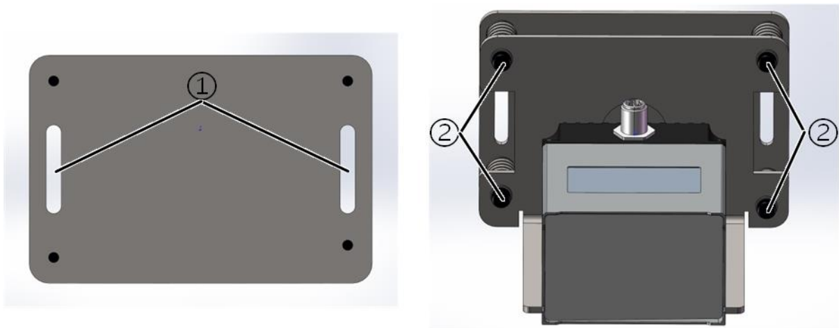
图 4.2: 可调支架安装
